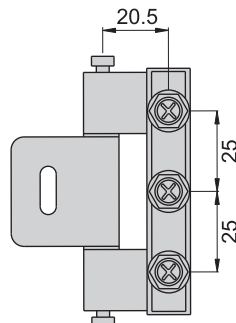
安装示意图
