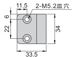
702#-1(B)
