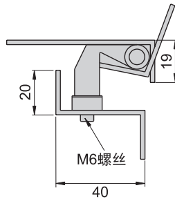
安装示意图
