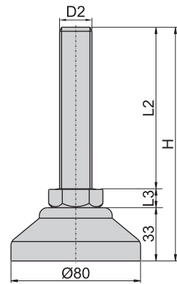
DS80 & D80 无防滑橡胶盘垫
