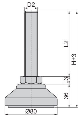
DS80P & D80P 配加防滑橡胶盘垫
